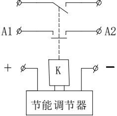
电路原理图
