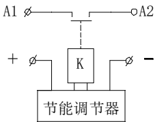
电路原理图
