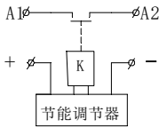
电路原理图
