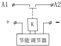
电路原理图
