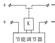
电路原理图
