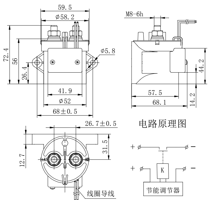
电路原理图
